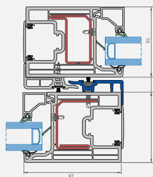
Coupe horizontale
