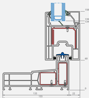
Coupe verticale
