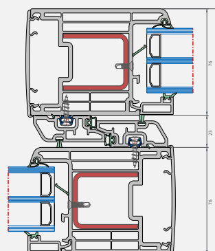
Coupe horizontale
