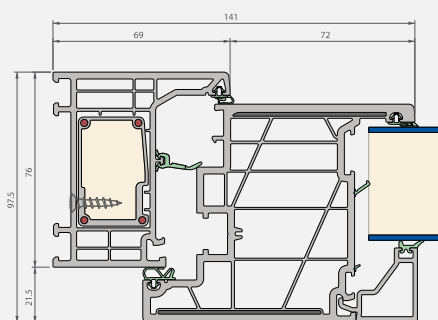
Coupe horizontale
