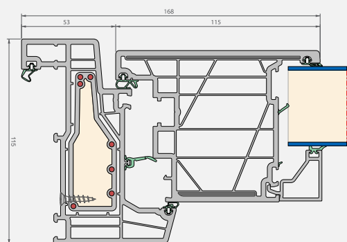
Coupe horizontale
