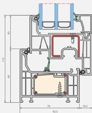
Coupe verticale
