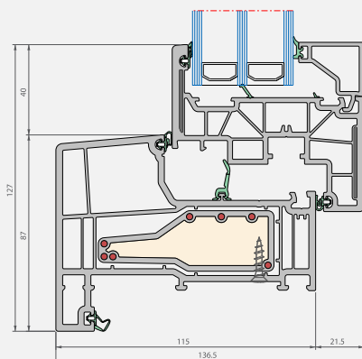
Coupe verticale
