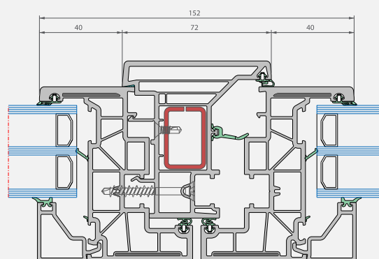
Coupe horizontale
