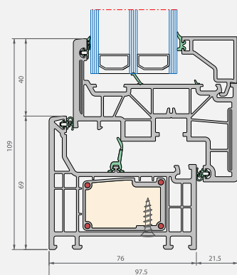
Coupe verticale
