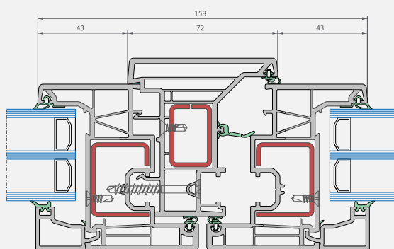
Coupe horizontale
