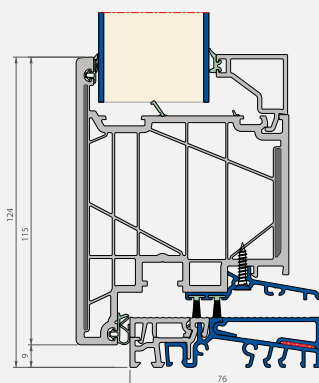
Coupe verticale
