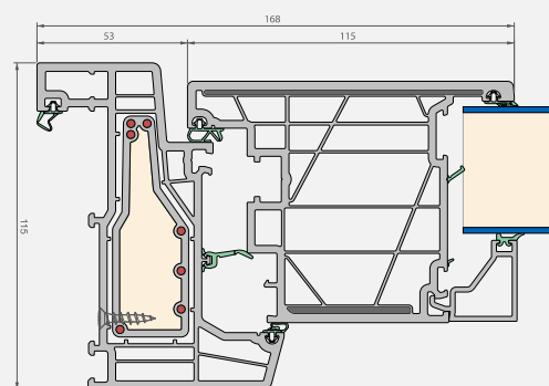
Coupe horizontale
