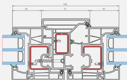
Coupe horizontale
