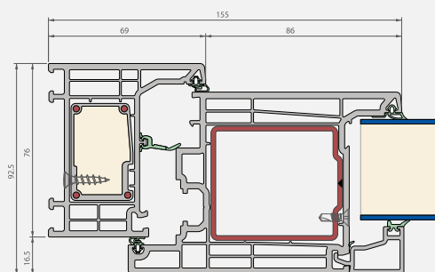
Coupe horizontale
