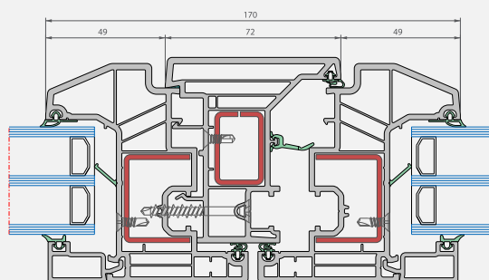
Coupe horizontale
