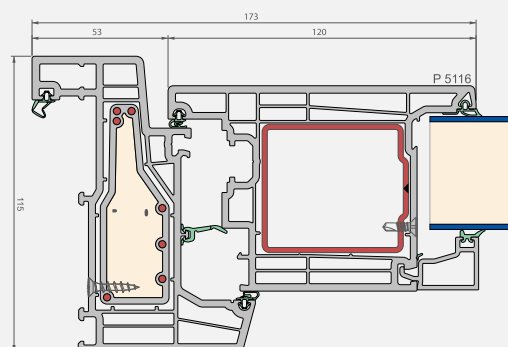
Horizontale snede
