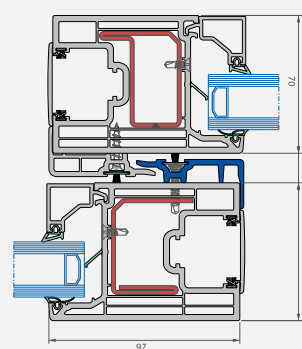
Horizontale snede
