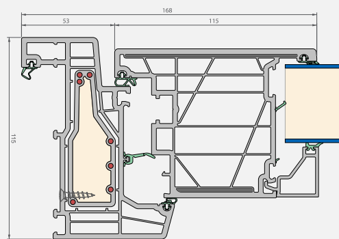
Horizontale snede
