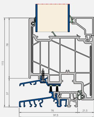
Verticale snede
