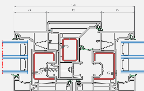
Horizontale snede
