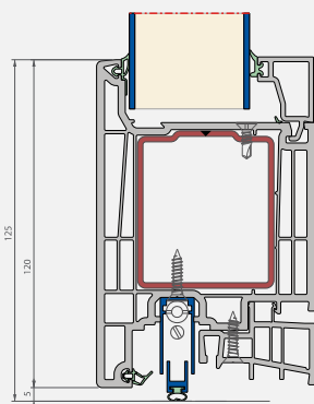
Verticale snede
