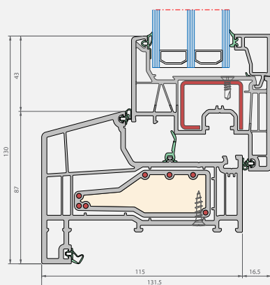
Verticale snede
