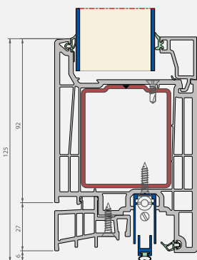
Verticale snede
