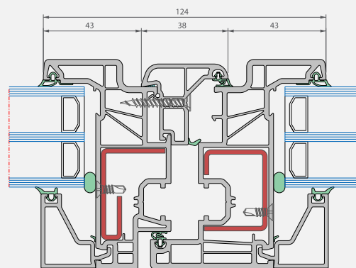
Horizontale snede
