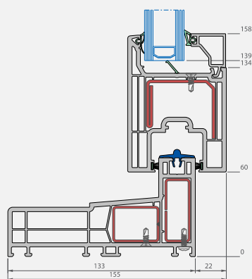
Verticale snede
