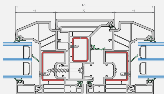
Horizontale snede
