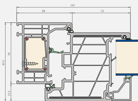
Horizontale snede
