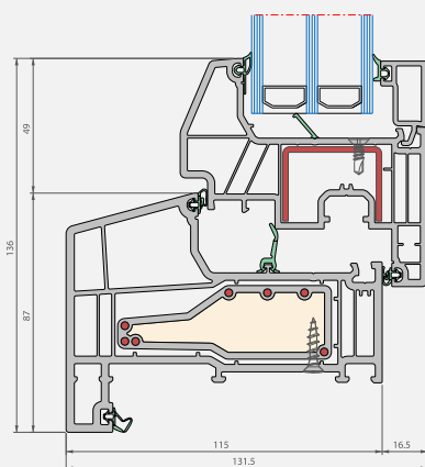
Verticale snede
