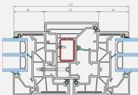
Horizontale snede
