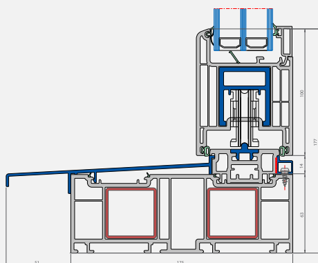
Verticale snede
