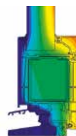
Tok izoterm Izračun v skladu z normo ISO 10077-2 s polnilom 36 mm
