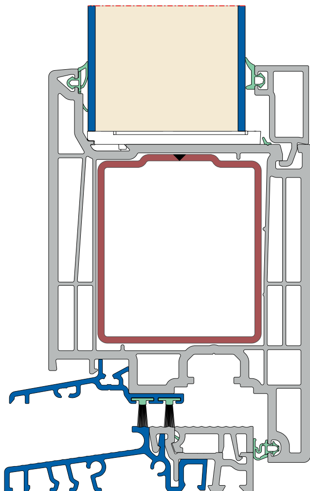
Sistem vhodnih vrat Elegant Infinity 76, prag in krilo Merilo: 1:1
