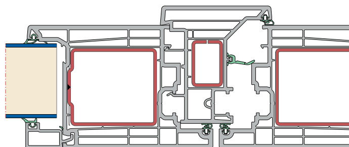
Sistem vhodnih vrat Elegant Infinity 76, srednji del štulpa Merilo: 1:2
