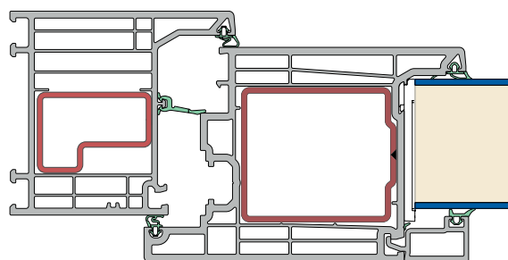
Sistem vhodnih vrat Elegant Infinity 76, okvir in krilo Merilo: 1:2
