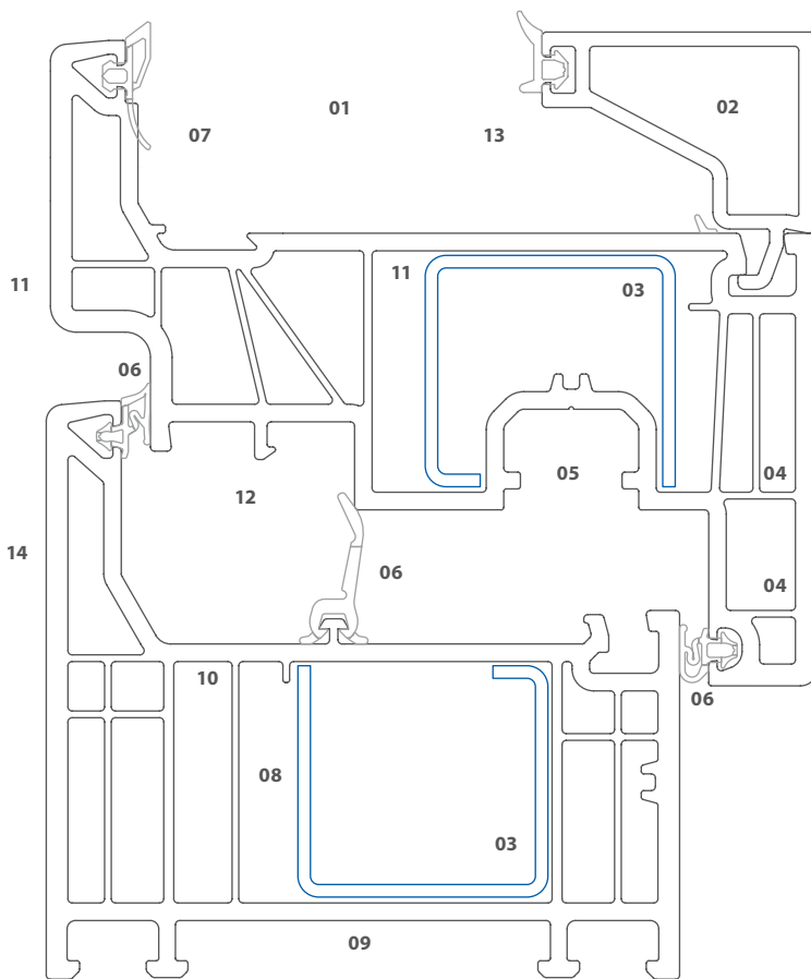
Elegant, premium krilo Okvir in krilo v isti ravnini Merilo: 1:1
