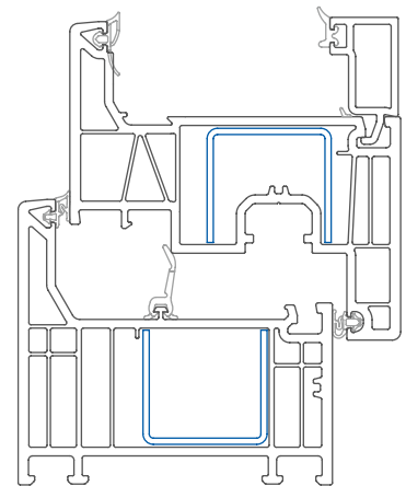
Elegant ravno krilo Okvir in krilo v zamaknjenih ravninah Merilo: 1:2
