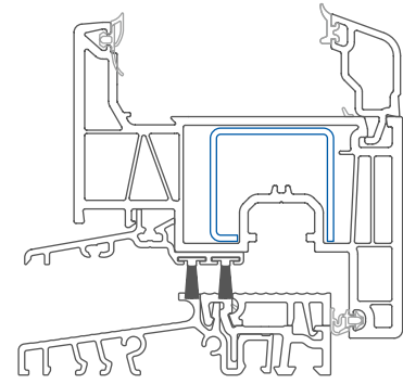
Elegant balkonska vrata z zaobljeno steklitveno letvico Merilo: 1:2
