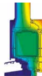
Tok izotermi Kalkulacija u skladu s normom ISO 10077-2 sa punjenjem od 36 mm
