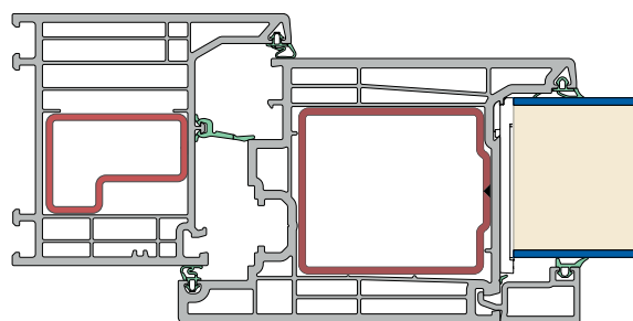
Sistem ulaznih vrata Elegant Infinity 76, okvir i krilo Merilo: 1:2
