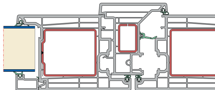
Sustav ulaznih vrata Elegant Infinity 76, srednji dio štulpa Mjerilo: 1:2
