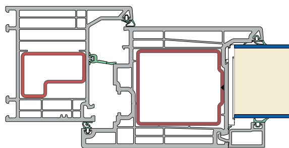
Sustav ulaznih vrata Elegant Infinity 76, okvir i krilo Mjerilo: 1:2
