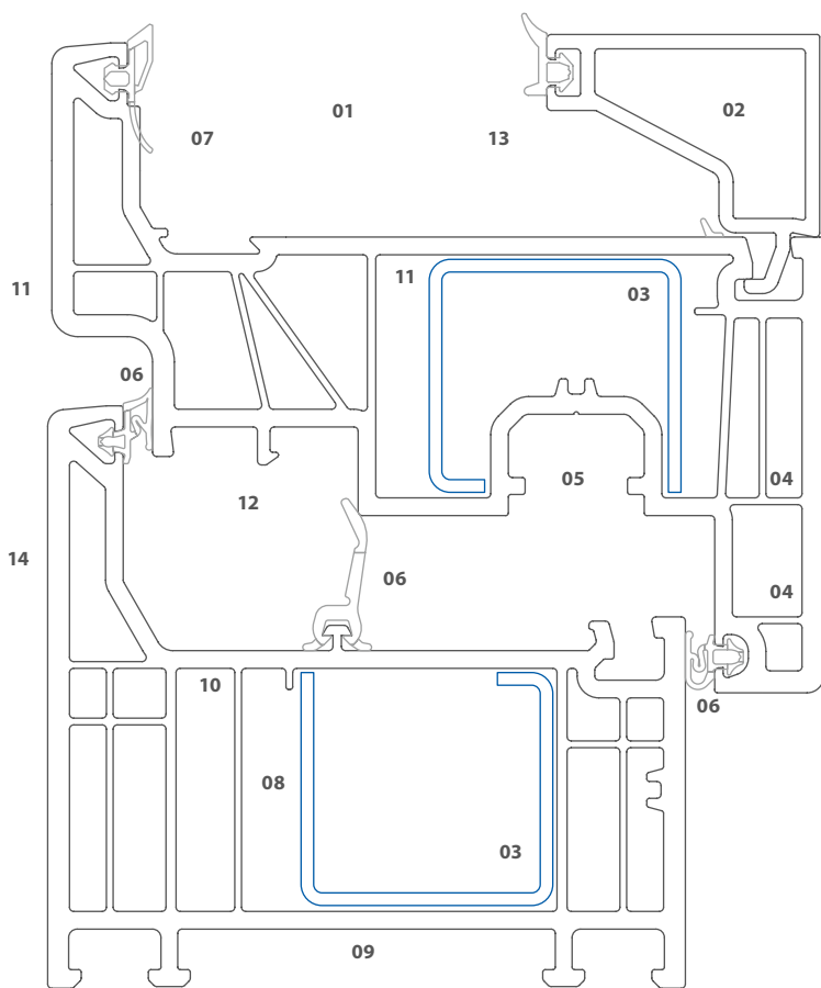
Elegant premium krilo Okvir i krilo u istoj ravni Mjerilo: 1:1
