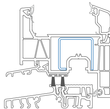
Elegant balkonska vrata sa pragom sa zaobljenom letvicom zastakljivanja Mjerilo: 1:2
