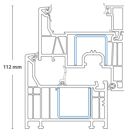
Elegante egyenes szárnyú változat Ábra: 1 : 2
