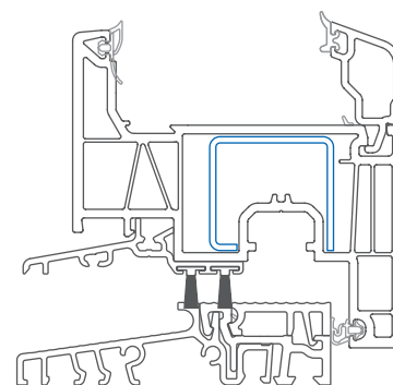
Elegantní práh balkonových dveří se šikmou zasklívací lištou · Obr.: 1 : 2
