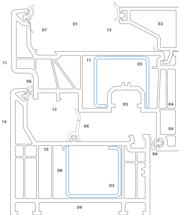
Elegante – varianta s předsazeným křídlem Obr.: 1 : 1
