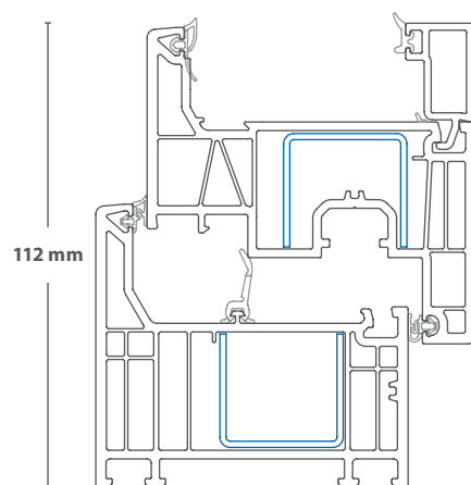
Elegante – varianta s rovným křídlem Obr.: 1 : 2
